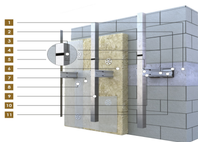
Вид - А
