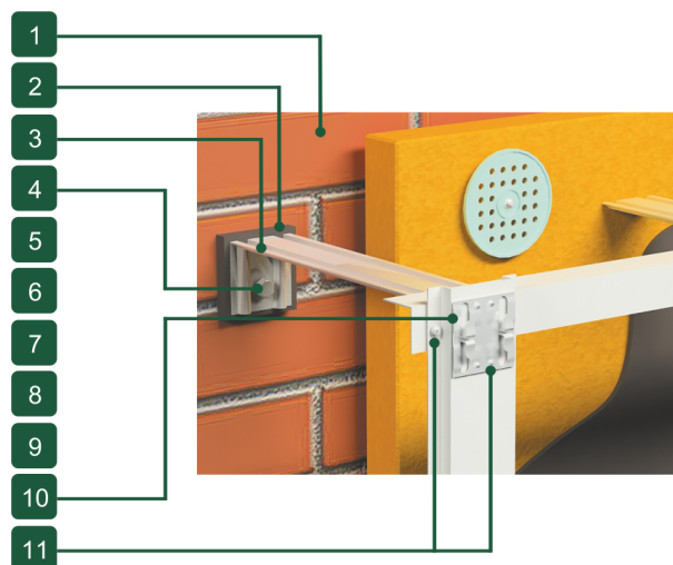
Узел крепления
