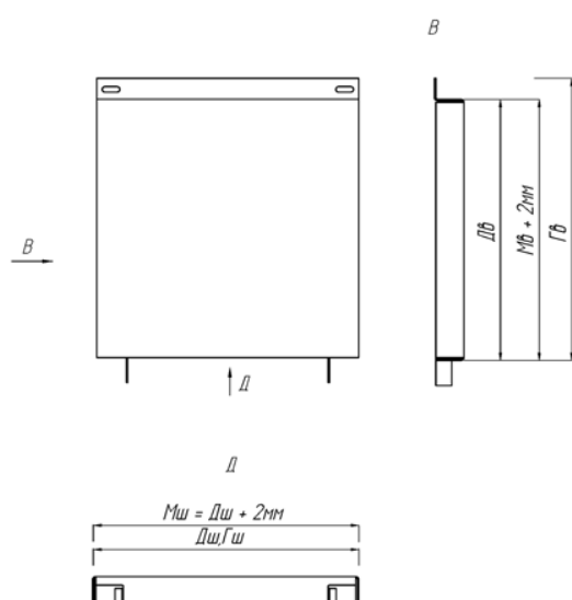
Прямоугольная кассета АЛГА 4000
