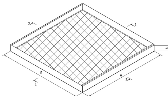
Общий вид панели MESH BOARDBOX
