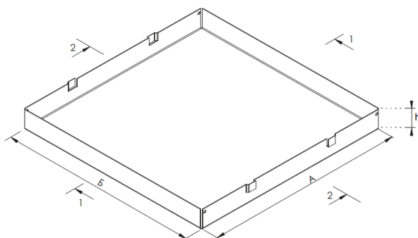
Общий вид панели CASSETTE HOOK-ON 300
