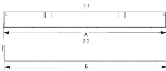
Основные параметры панели CASSETTE HOOK-ON 300
